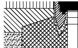
Versetzen und Vergiessen
